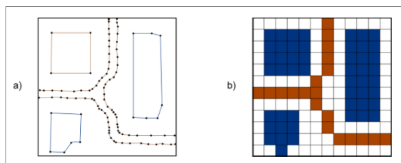
Ilustración 1. Modelos de representación Comparación del modelo vectorial (a) y el ráster (b) Fuente: Olaya, 2016
